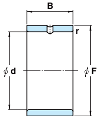
JR ..JS1
